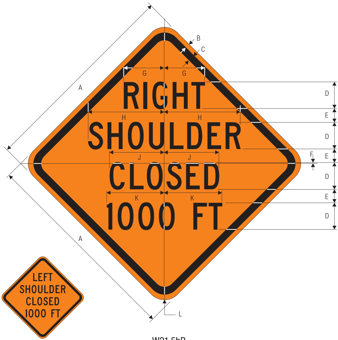
W21-5bL
