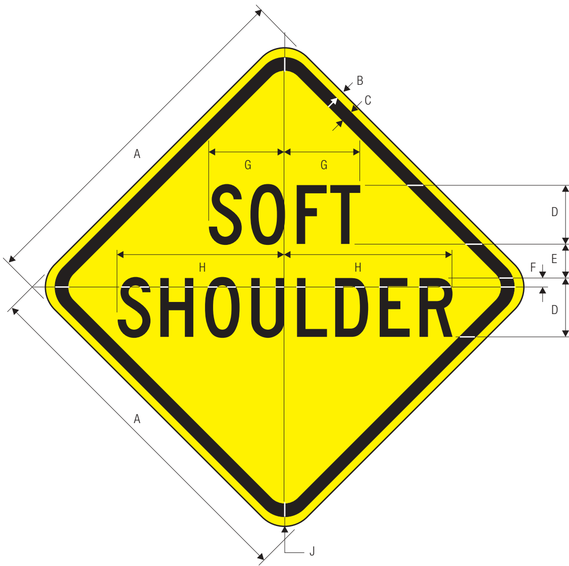
W8-4
