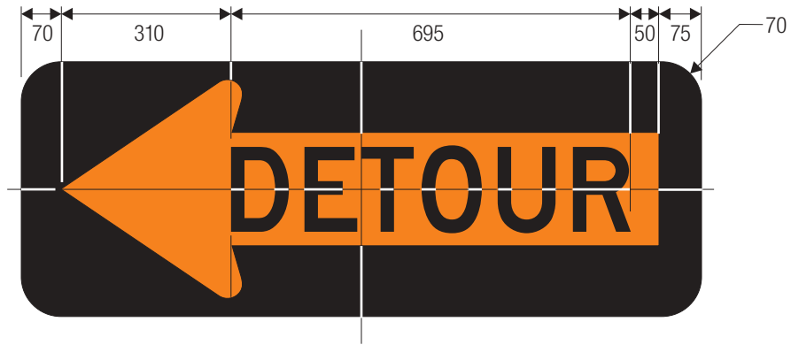
M4-10L
