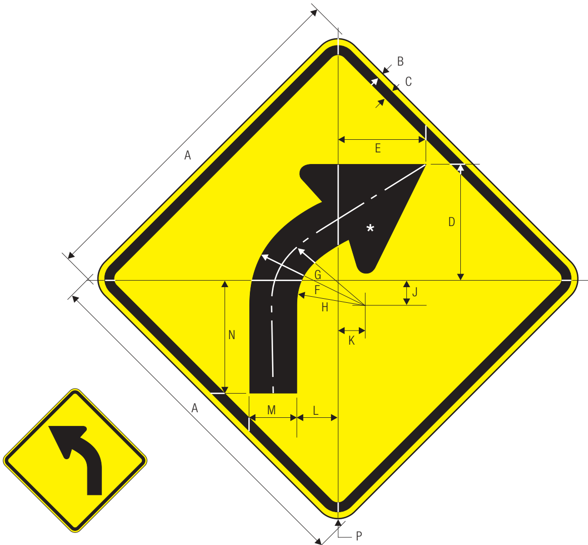
W1-2L
