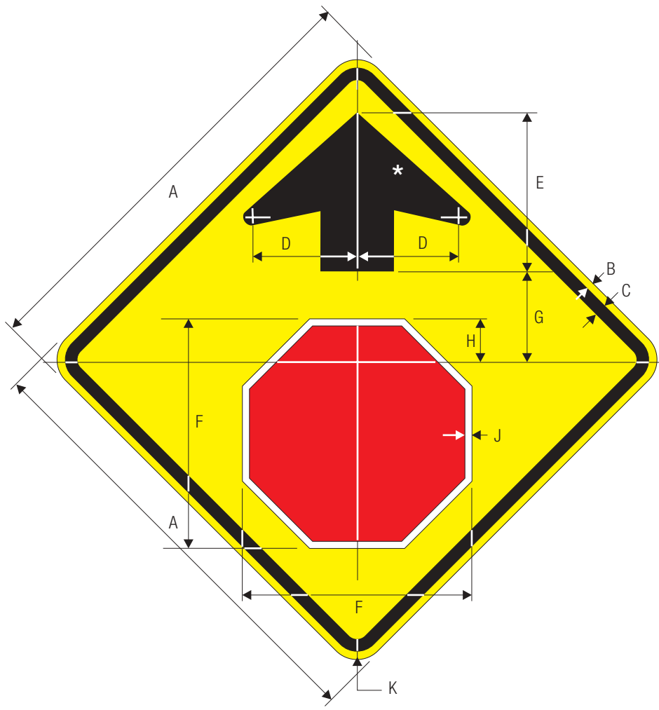
W3-1a
