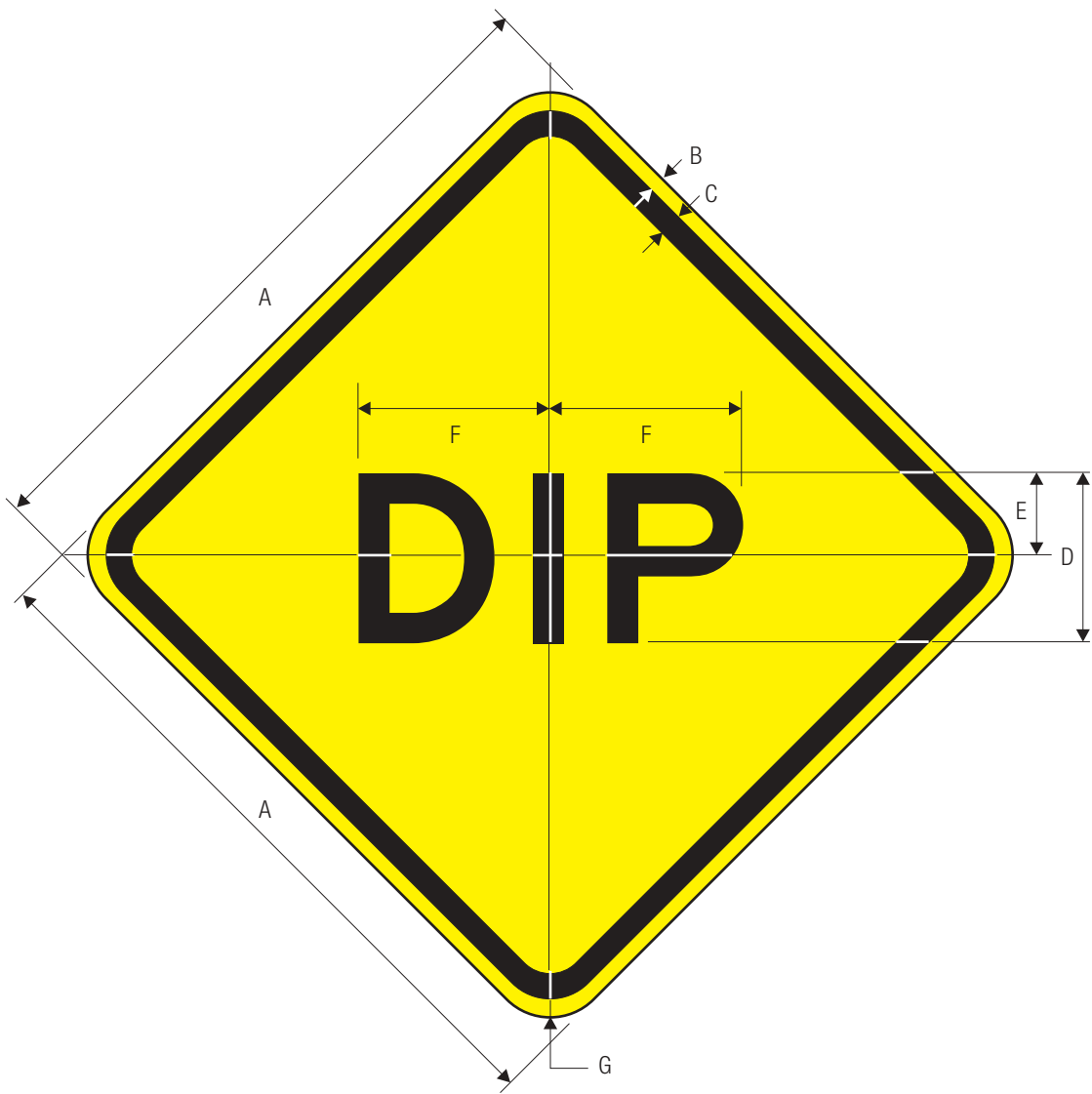
W8-2
