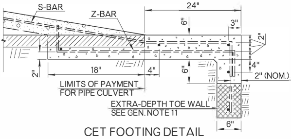
CET FOOTING DETAIL
