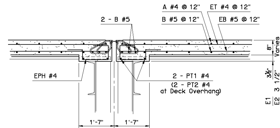
SECTION E1 AND E2
