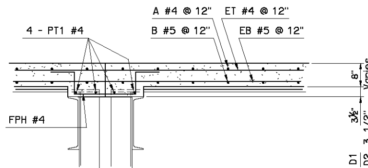
SECTION D1 AND D2
