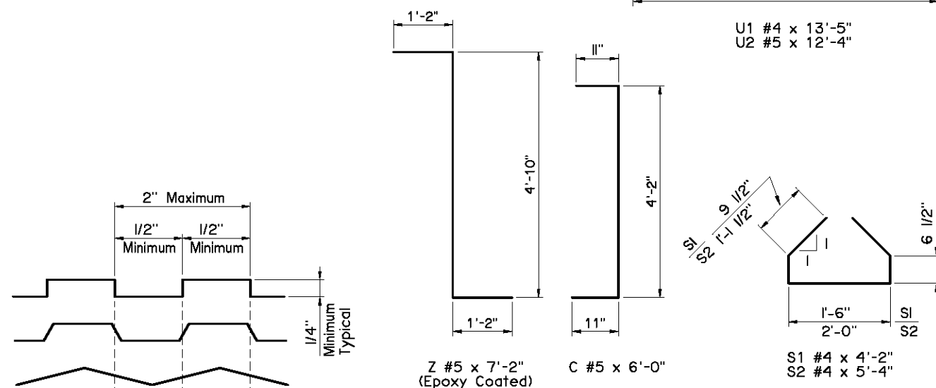
TYPE IV P.C. BEAMS
