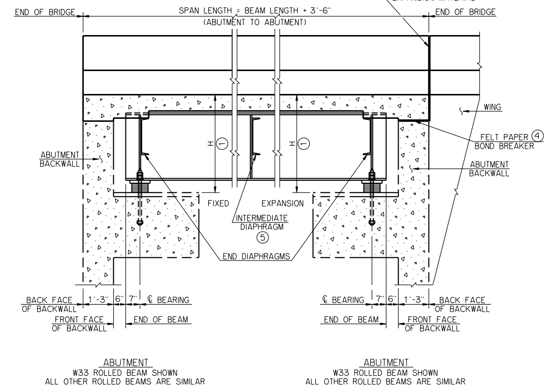
LONGITUDINAL SECTION
