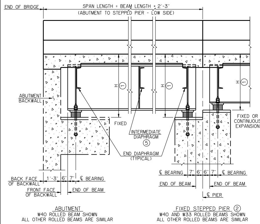
LONGITUDINAL SECTION
