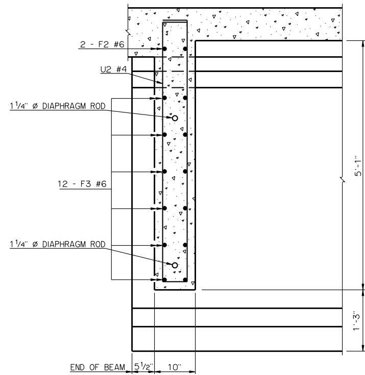
SECTION A-A
