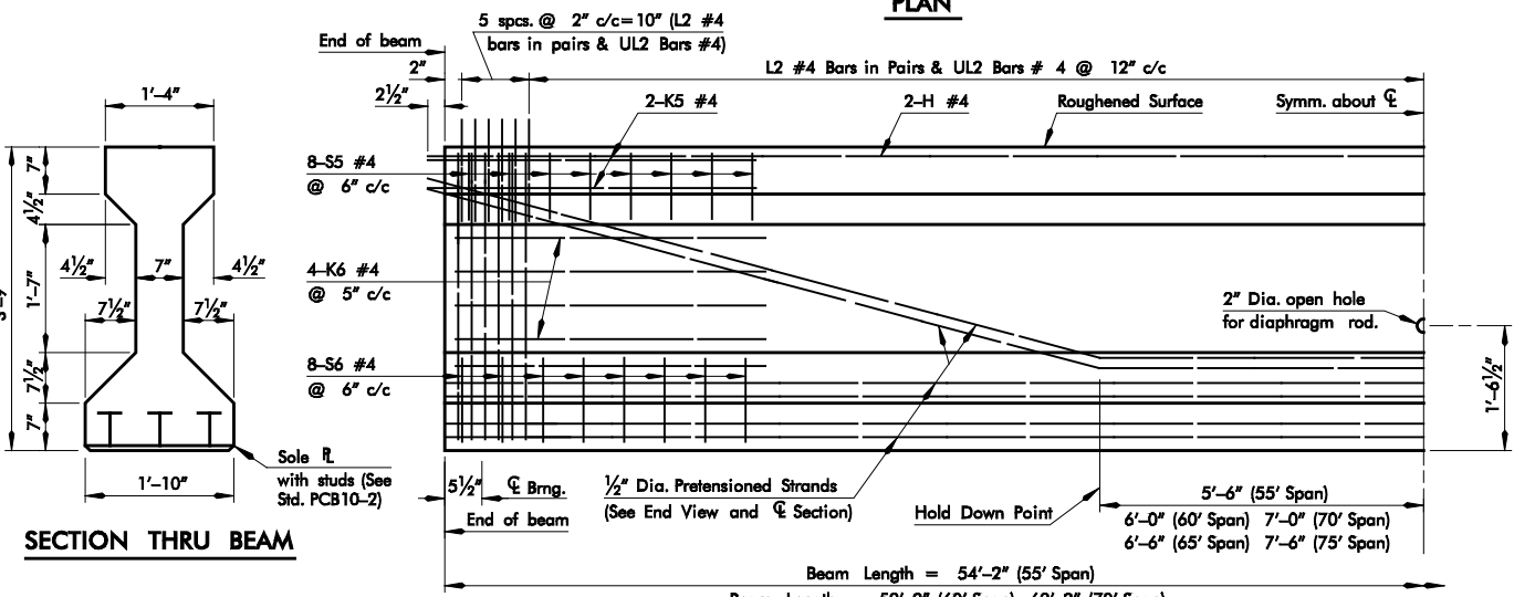
ELEVATION - 0° SKEW
